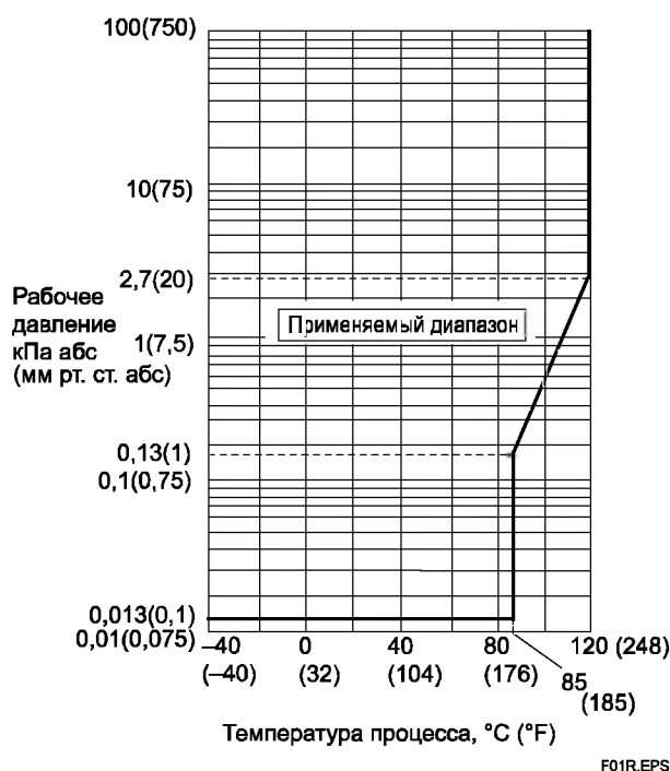
Рисунок 1-1. Рабочее давление и температура процесса [для модели EJX610A]
