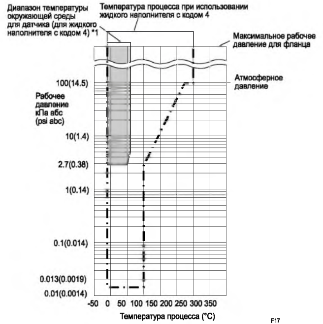
Рисунок 1-5. Рабочее давление и температура процесса (Жидкий наполнитель: силиконовое масло для использования в среде глубокого вакуума)
