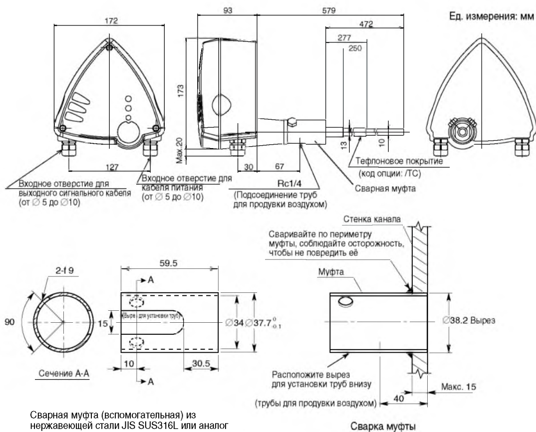
Размеры датчика запыленности DT450G (Модель с муфтовым креплением)
