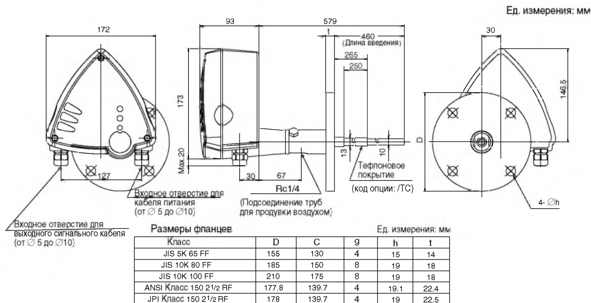
Размеры датчика запыленности DT450G (модель с фланцевым креплением)
